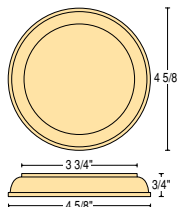
C-7317 Rosette
