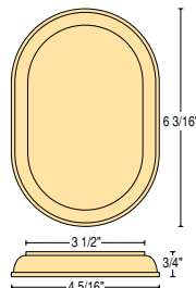
C-7237 Rosette
