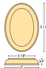
C-7337 Rosette
