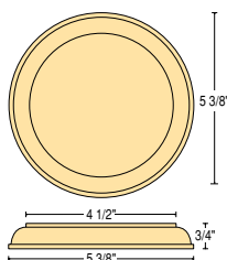
C-7217 Rosette
